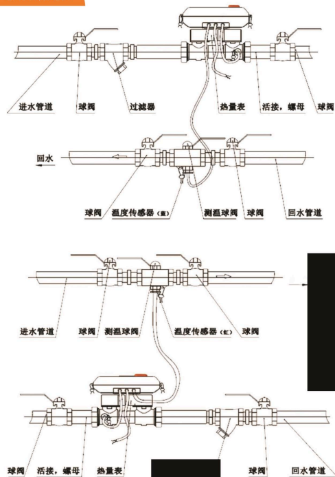
进回水安装示意图
